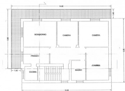
PIANO PRIMO
